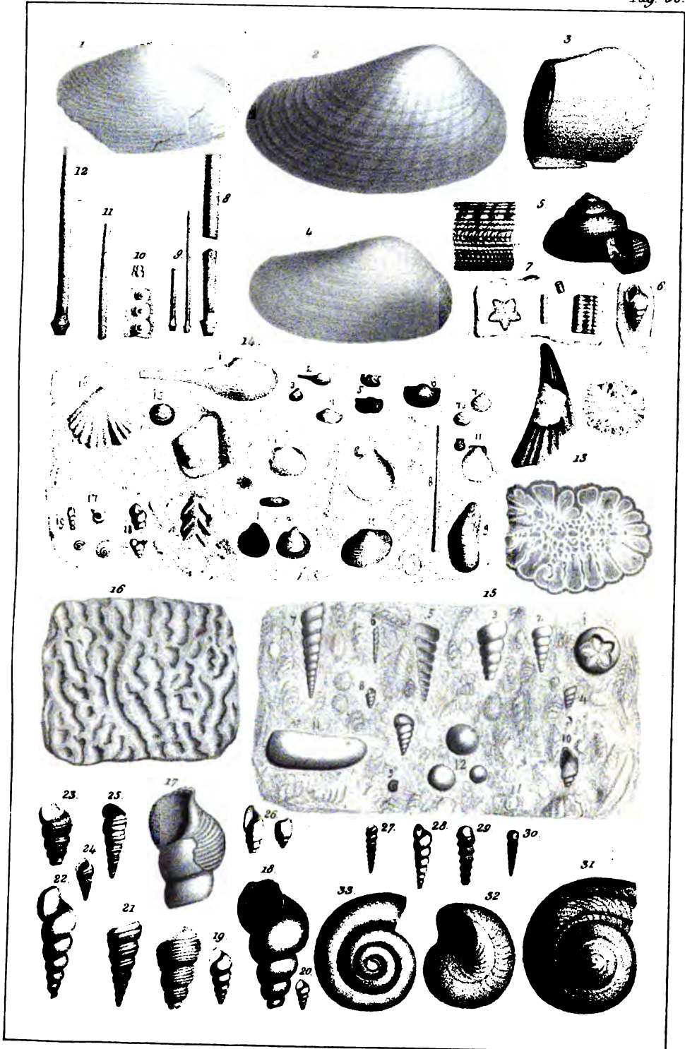
Ozenstedt, Jura!
